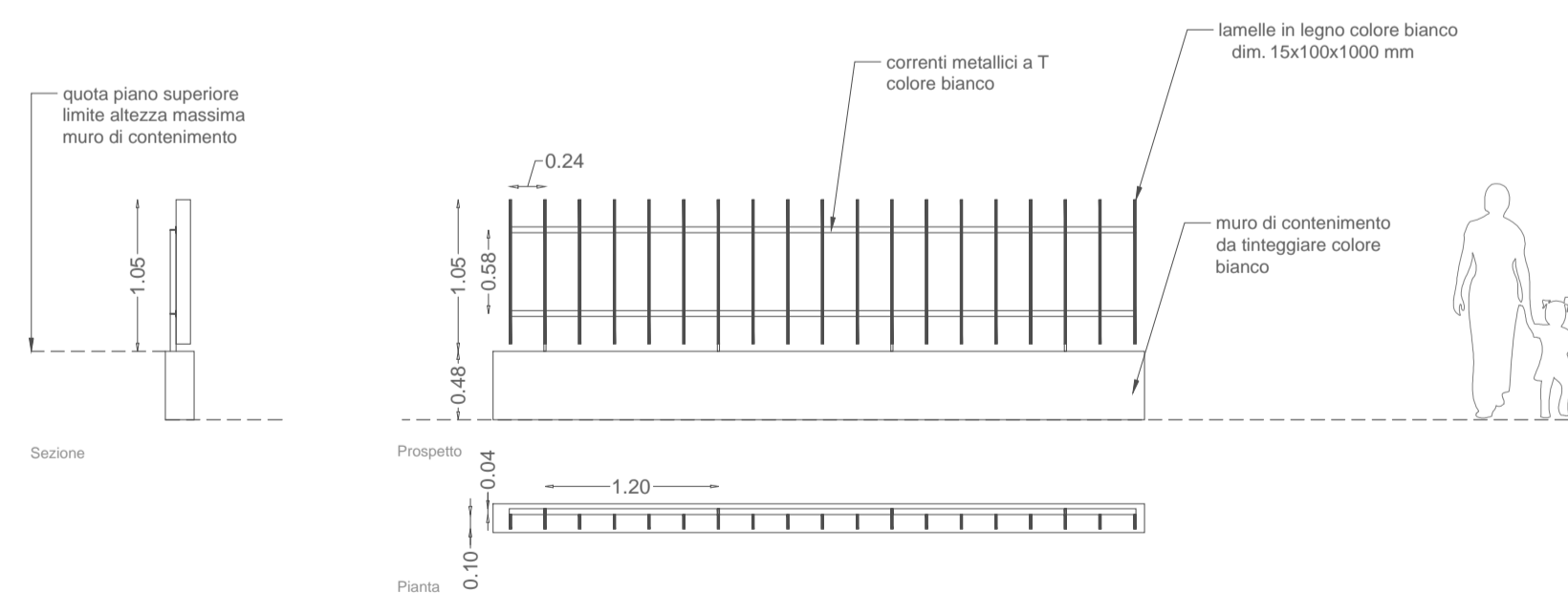
RECINZIONE scala 1:50
